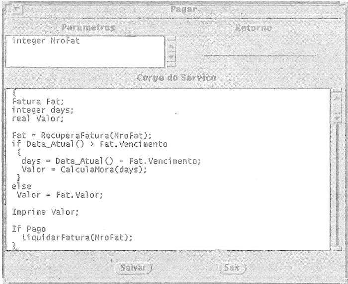
Figura 9 - Janela do serviço Pagar
