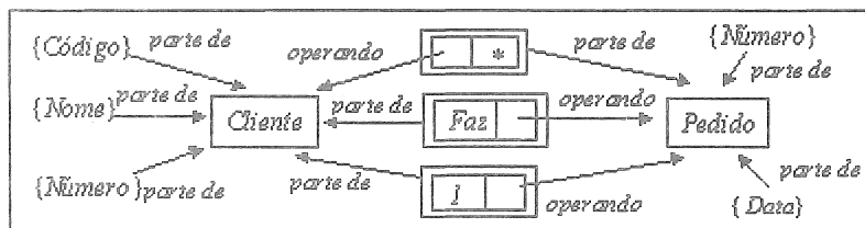
Figura 13 - Descrição RC do Modelo de Objetos do método Fusion
