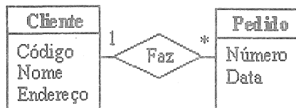
Figura 14 - Modelo de Objetos do método Fusion
