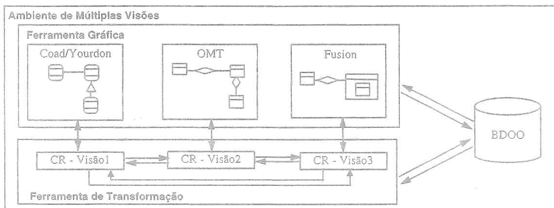
Figura 1 - Arquitetura geral do ambiente
