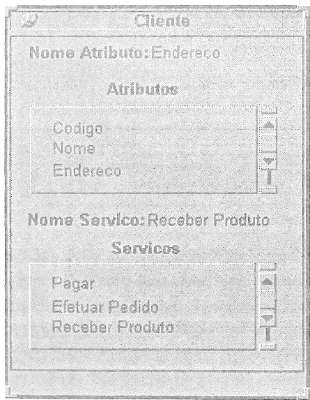
Figura 8 - Janela de elementos para a classe Cliente
