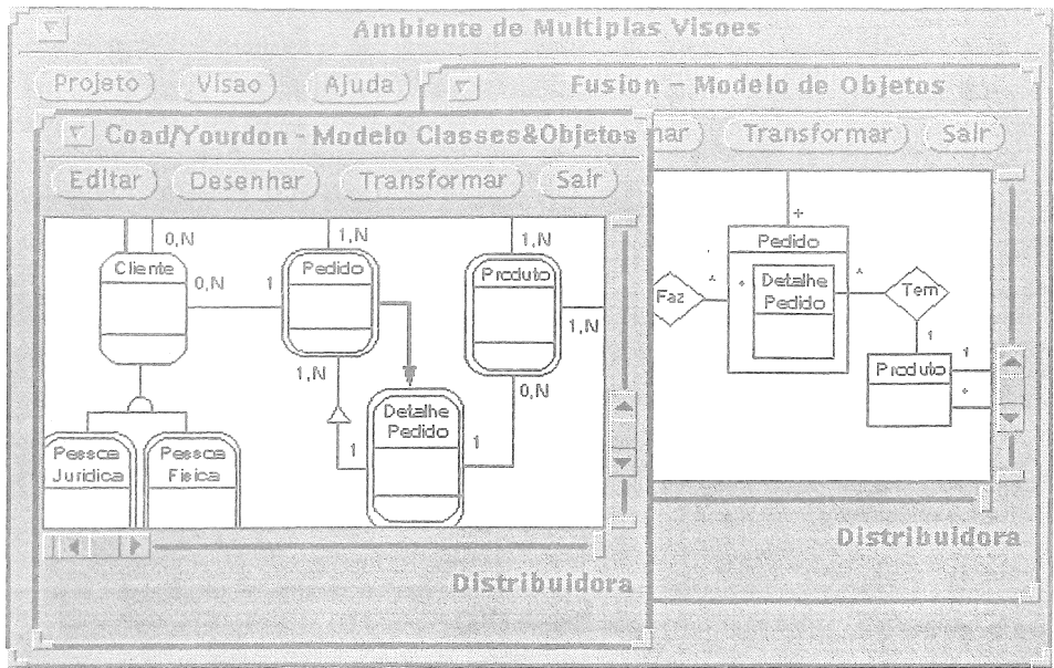
Figura 7 - Visão geral da Ferramenta Gráfica
