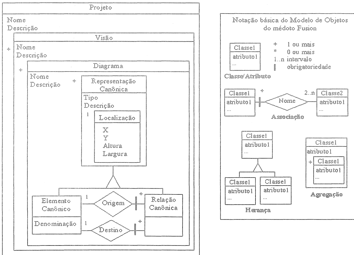
Figura 4 - Metamodelo para persistência das visões
