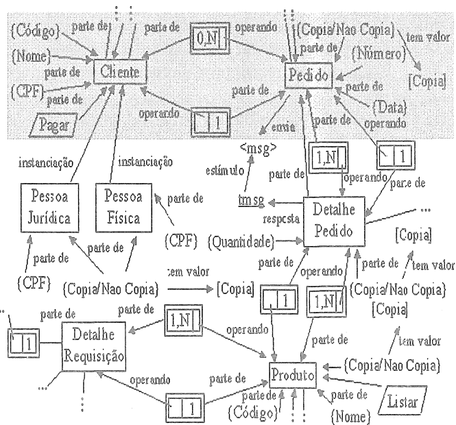
Figura 3 - Parte da descrição RC do Modelo Classes&Objetos do método Coad/Yourdon
