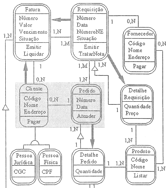
Figura 2 - Modelo de Classes&Objetos do método de Coad/Yourdon
